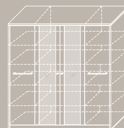
L 0138 187x45x192h
